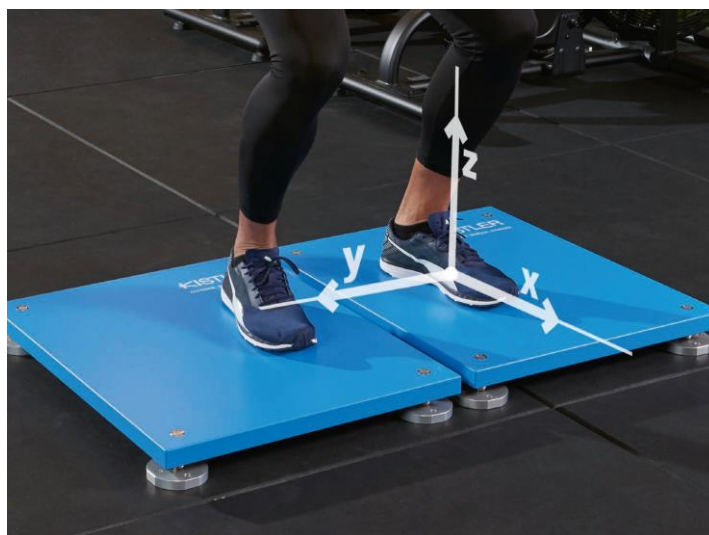
Рис. 1. Система 3D видеорегистрации и анализа движений спортсмена «Qualisys Motion Capture» с синхронизированной платформой «Kistler»:
